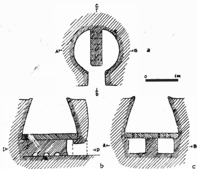
Fig. 16. — Cuptor de olar, cultura Cucuteni, faza Cucuteni B (așezarea Glăvăneștii Vechi).
