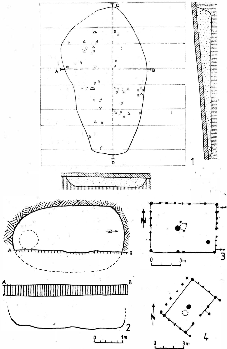
Fig. 35. — Tipuri de locuințe din epoca neolitică. A. Cultura Dudești, groapă de bordei, de la Cleanov-„Fiera”; B. Cultura Boian. 2. Groapă de bordei de la Bogata (faza Giulești); 3. Locuință de suprafață de la Tanglu (faza Vidra) și 4. Locuință de suprafață de la Petru Rareș (faza de tranziție).
